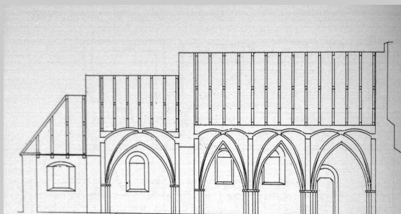
Svedala gamla kyrka, längdenomskärning enligt Brunius 1844.
